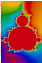
Mandelbrotin joukko
